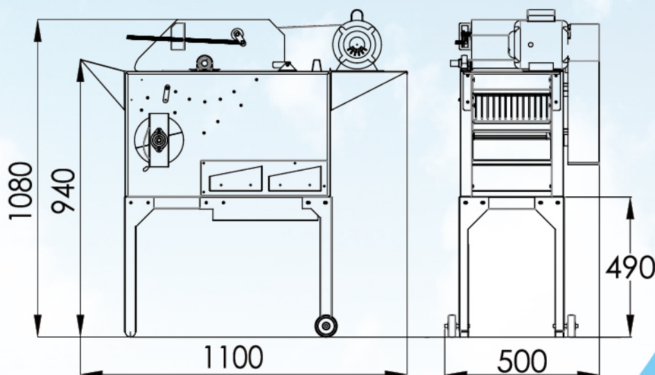
側視圖
